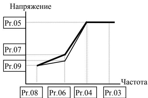
Кривая U/f для вентилятора/насоса
